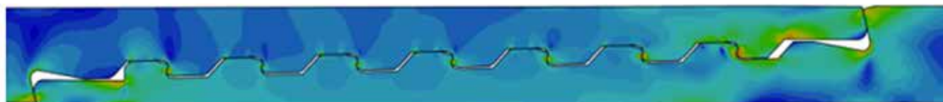
Figure 3 - Le S-Maxx répartit la précharge sur toute la longueur du filet, beaucoup plus facilement qu'un filet à départ unique.
