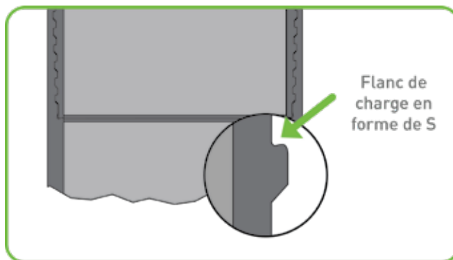
Figure 1 - Schéma du flanc de charge en forme de S du profil de filetage S-Maxx.
